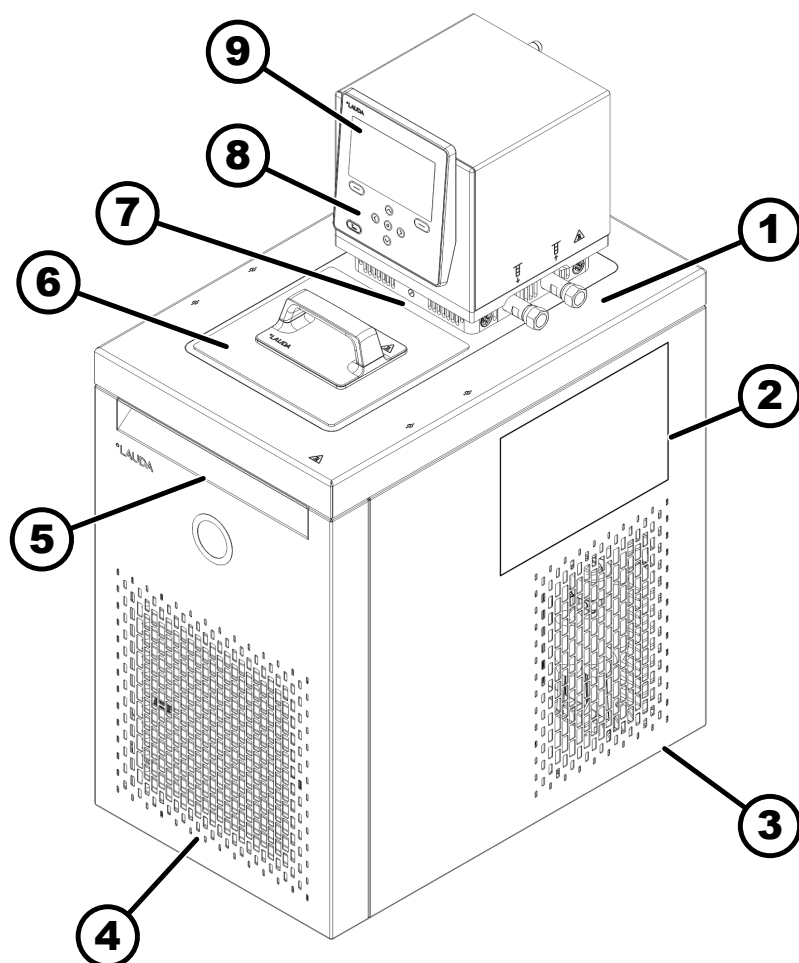
Fig. 7: Cryothermostat MAX, vue frontale
