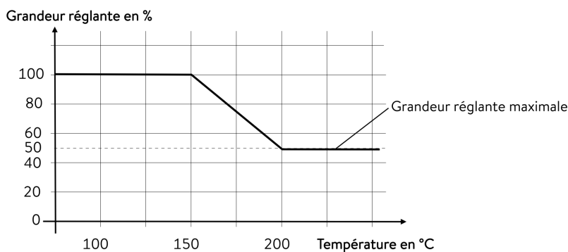
Fig. 67: Limitation dynamique de la puissance de chauffe
