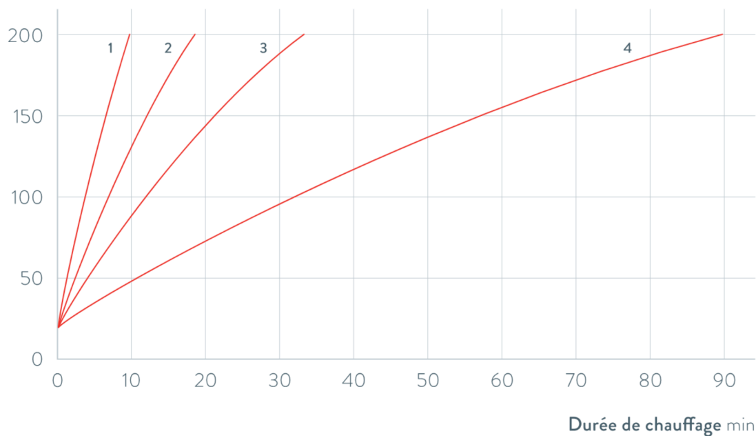
Fig. 80: Courbes de montée en température pour thermostats chauffants Universa PRO
