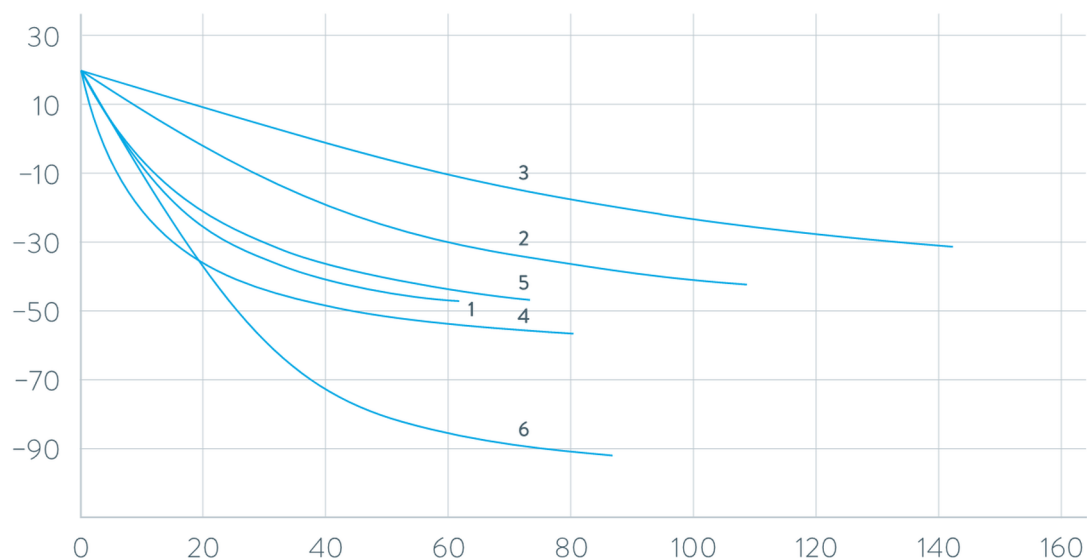
Fig. 83: Courbes de refroidissement pour cryothermostats Universa MAX
