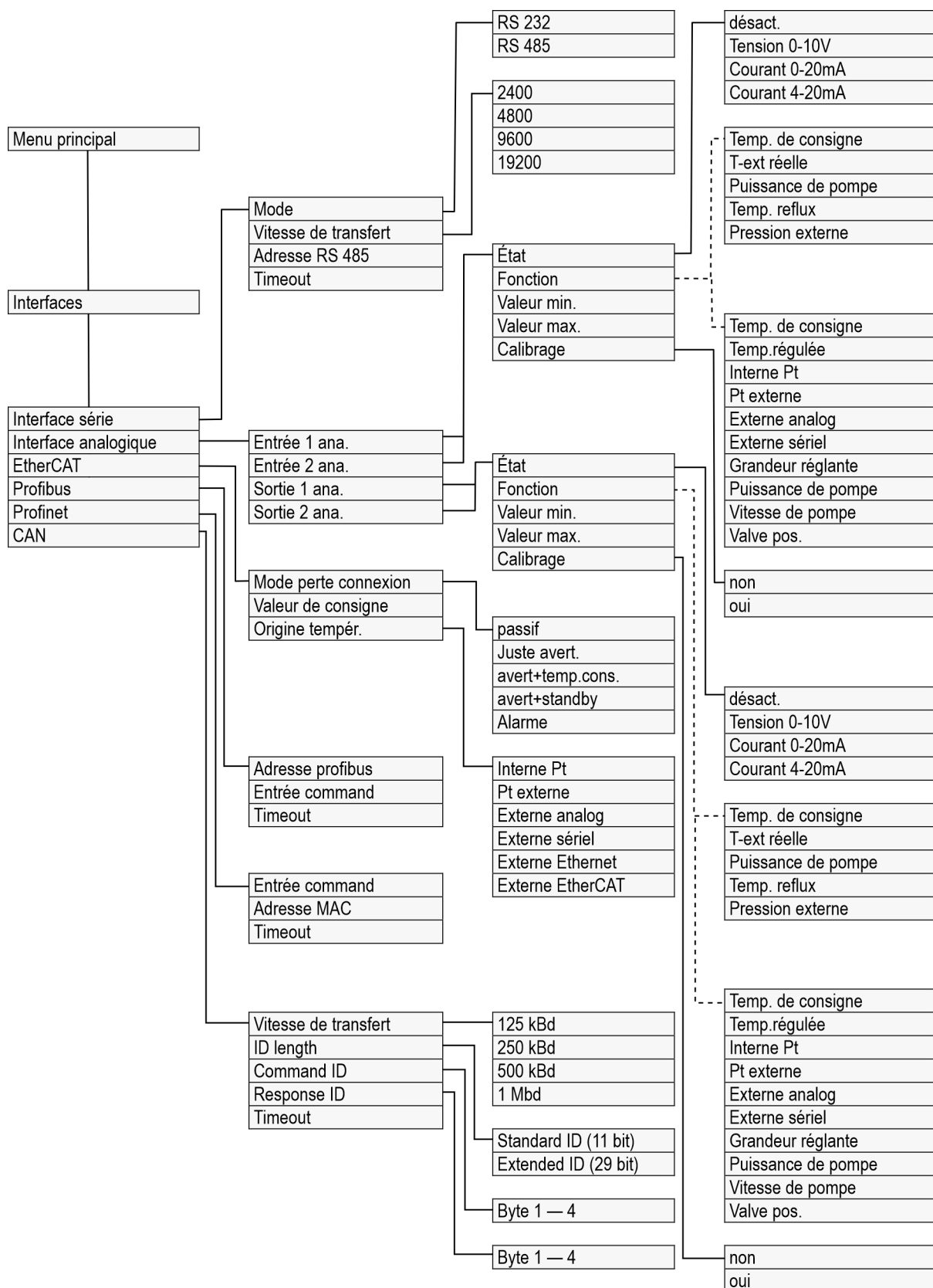
Fig. 57: Structure du menu partie 4, pour MAX et PRO
