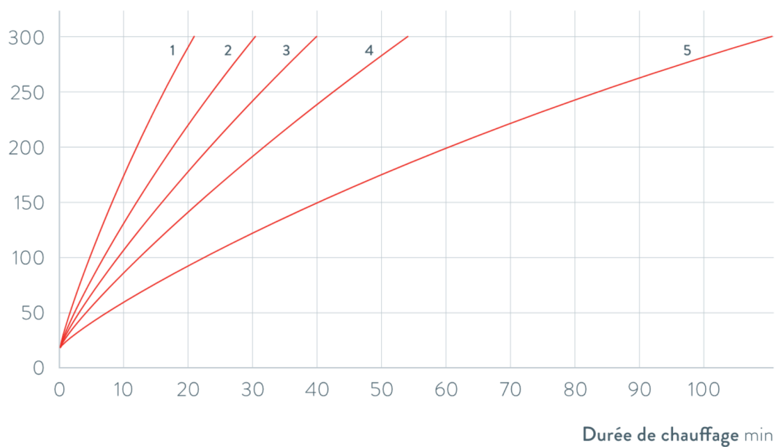
Fig. 81: Courbes de montée en température pour thermostats chauffants Universa MAX
